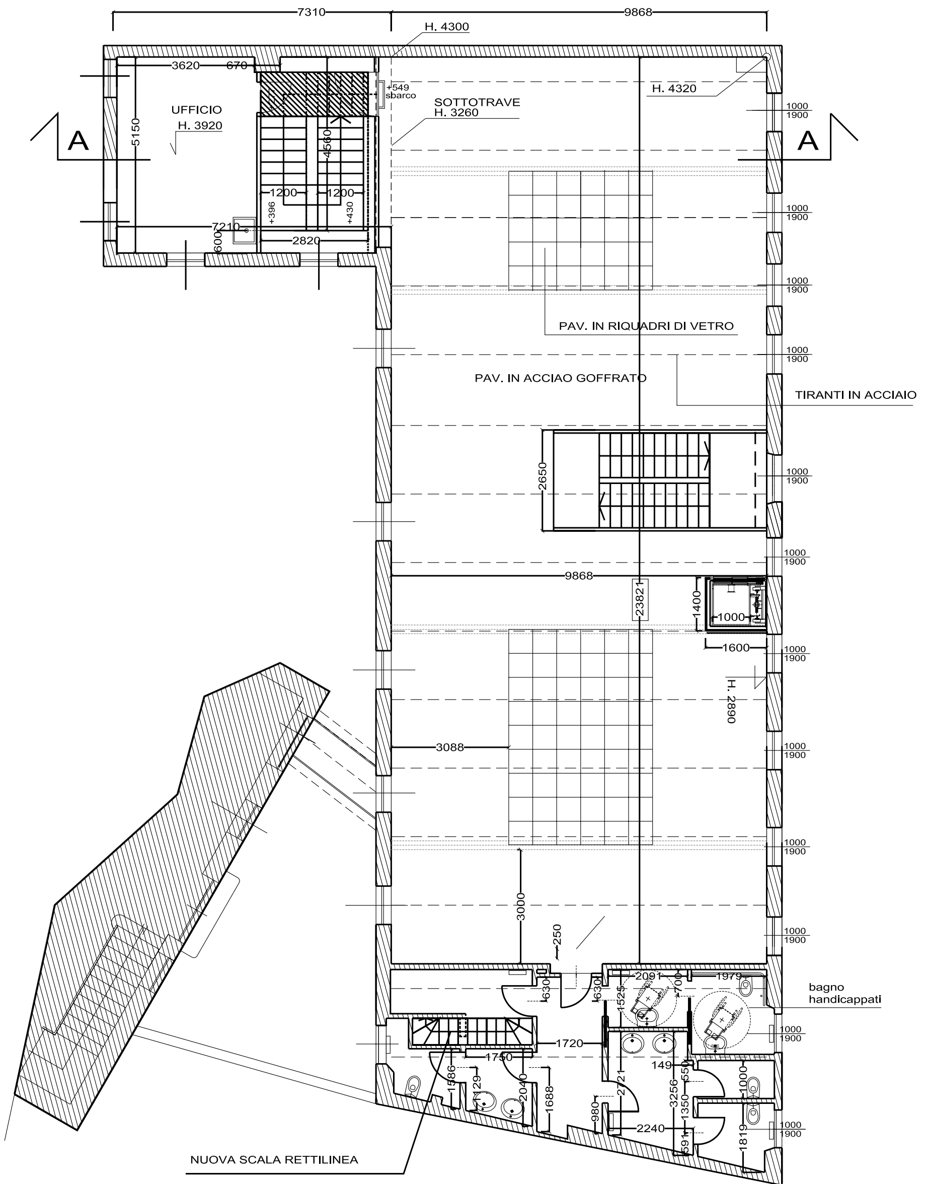
PLANIMETRIA - PIANO PRIMO
